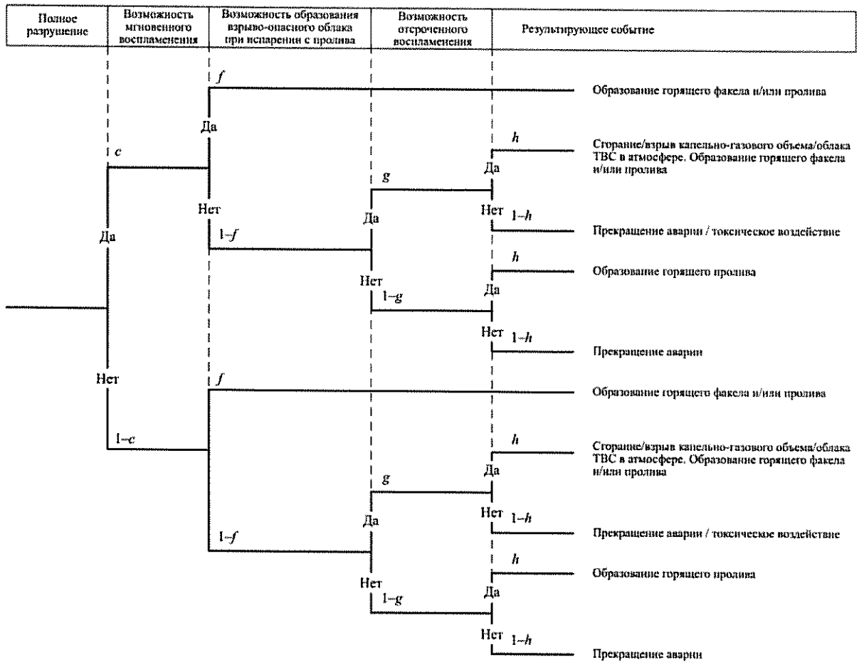
Рисунок 4-1. «Дерево событий» при разгерметизации технологического трубопровода на эстакаде
