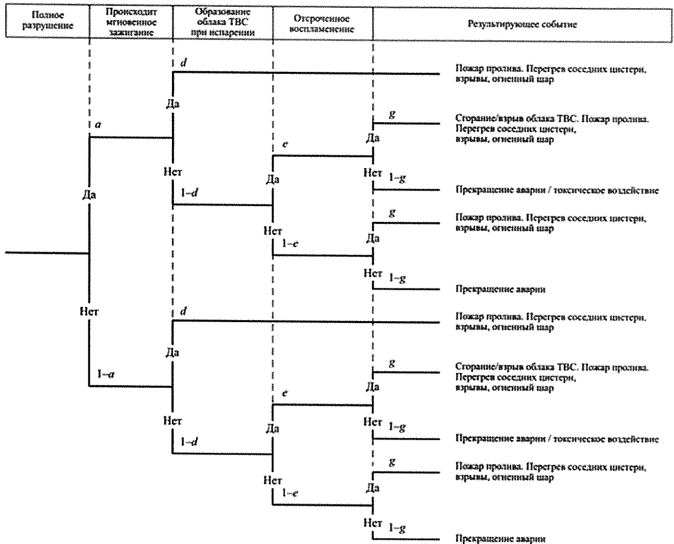
Рисунок 4-2. «Дерево событий» схода (разрушения) цистерны (группы цистерн), содержащей продукт при атмосферном давлении
