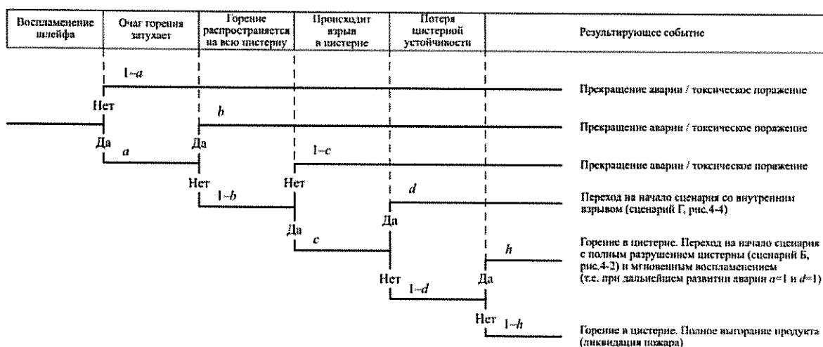
Рисунок 4-3. «Дерево событий» при выходе газовой фазы из цистерны (образование шлейфа паров взрывопожароопасной жидкости на дыхательной арматуре (люке, зазоре) и его зажигание с формированием очага горения)
