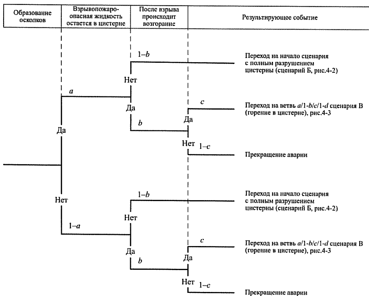
Рисунок 4-4. «Дерево событий» при взрыве внутри цистерны
