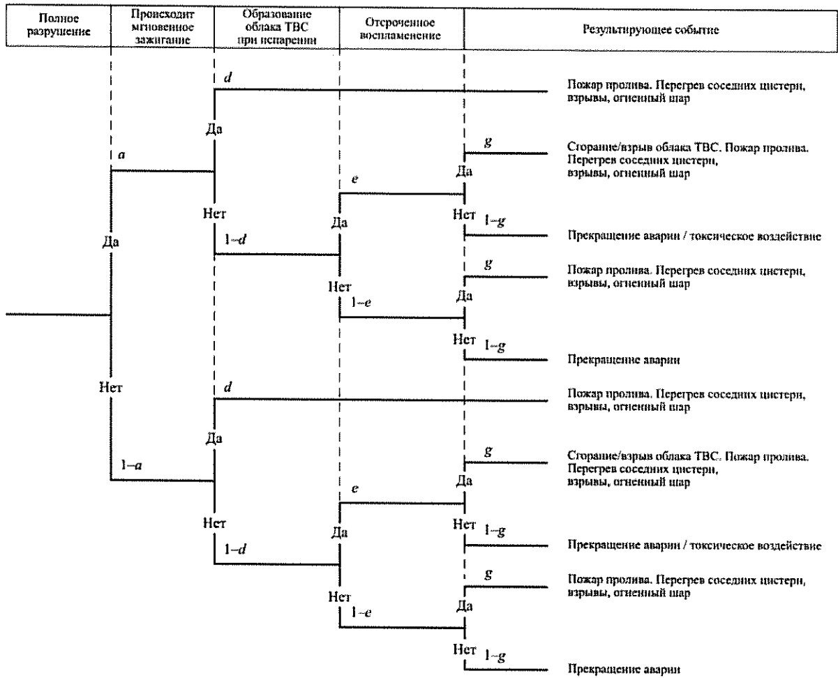
Рисунок 4-5. «Дерево событий» для сценария с воспламенением цистерны при сливе-наливе взрывопожароопасной жидкости
